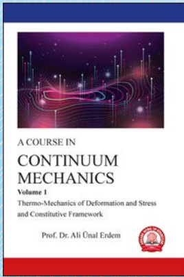
CONTINUUM MECHANICS Volume 1 Prof. Dr. Ali Ünal ERDEM
